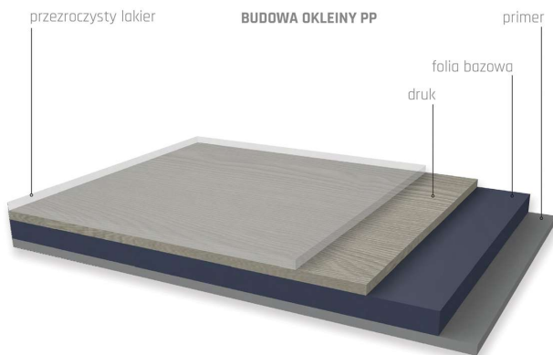
BUDOWA OKLEINY PP
