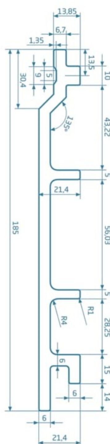
PROFIL ELEWACYJNY 185 X 20,4 MM
