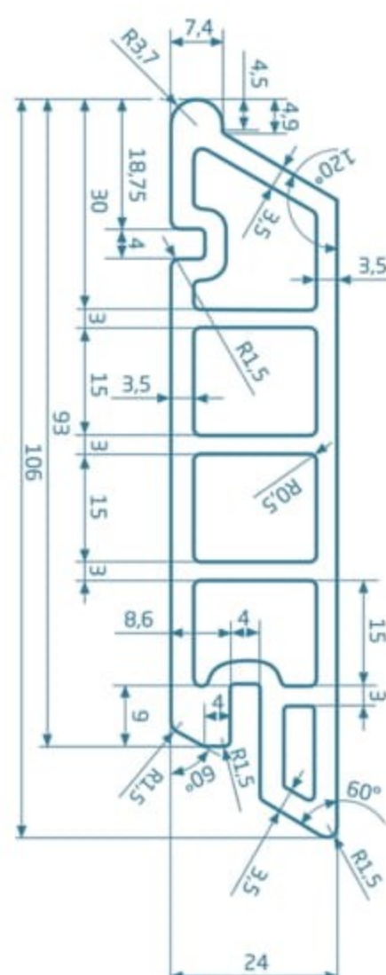
PROFIL ELEWACYJNY 106 X 24 MM
