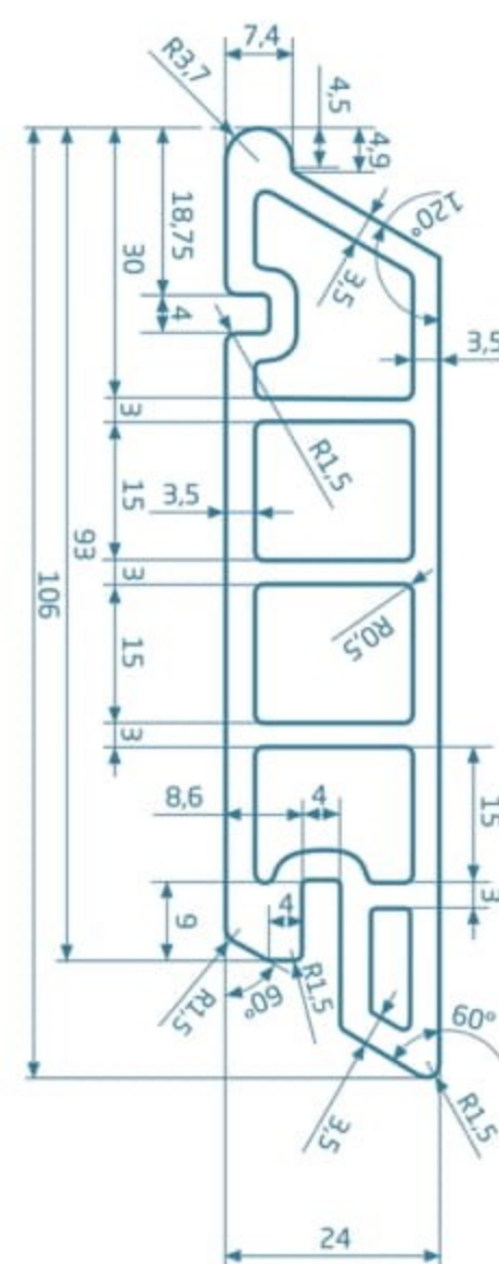
PROFIL ELEWACYJNY 106 X 24 MM
