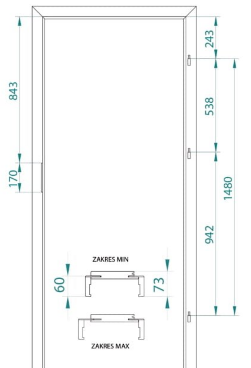
OŚCIEŻNICA REGULOWANA DO DRZWI PRZYLGOWYCH
