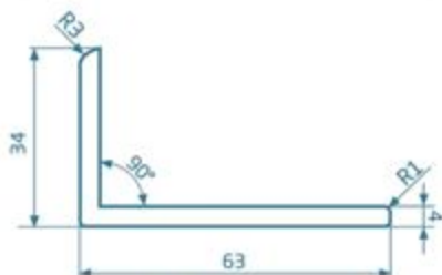
LISTWA WYKOŃCZENIOWA 34 X 63
